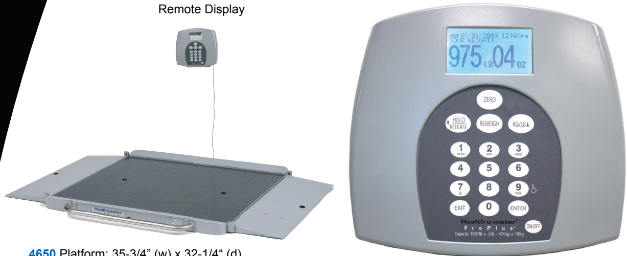
4650 Platform: 35-3/4" (w) x 32-1/4" (d) 4700 Extra Large Platform: 43" (w) x 42" (d)
